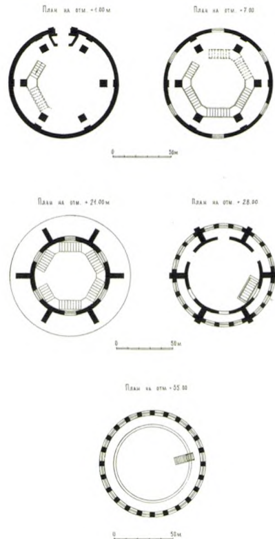
Планы башни на отметках 1,00, 7,00, 21,00, 28,00 и 35,00 м
