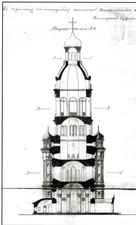
Колокольня. Разрез. Арх. А. Иваницкий, 1871 г. Из фондов Национального музея Республики Коми
