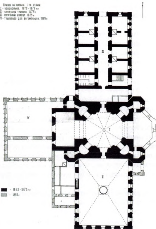
Храм-колокольня с примыкающими постройками. План на уровне 1-го этажа
